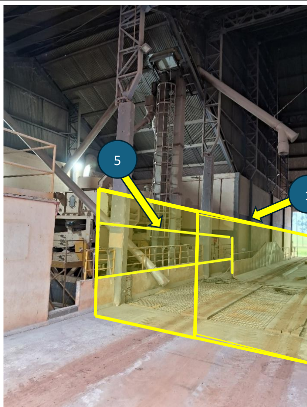
Figura 8 - Detalhe do portão e gradil a ser instalado.
