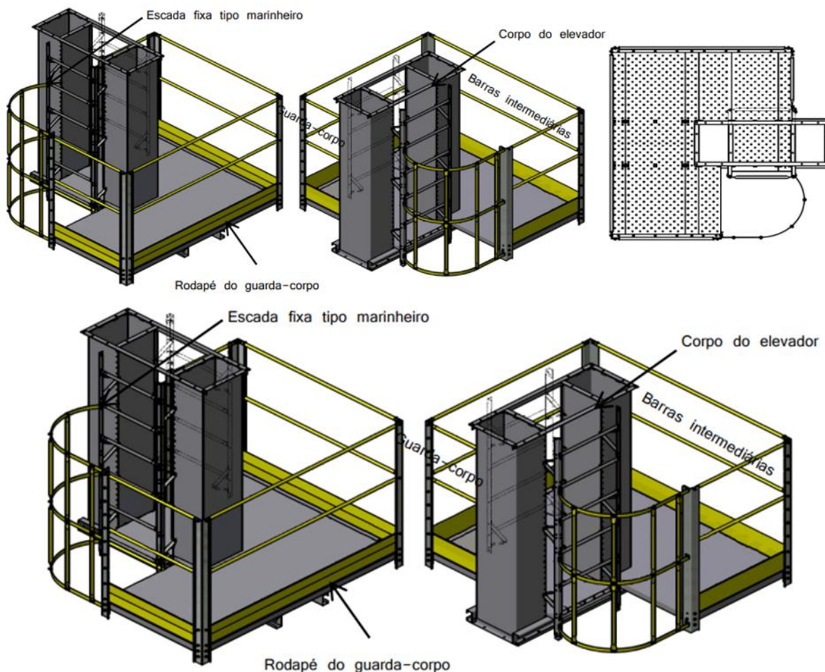
Imagem 81: Detalhe plataforma com quebra de fluxo.
