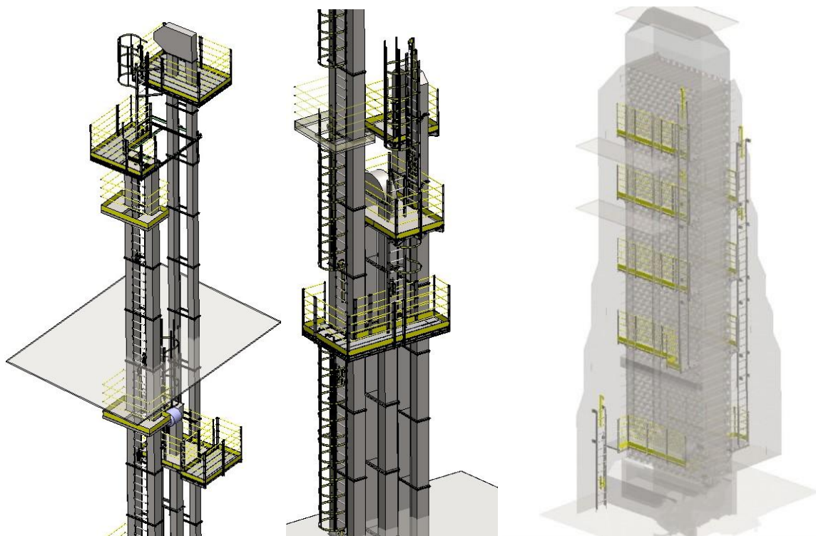
Imagem 87: Modelo de croqui para projeto inicial – Adequação de plataformas.
