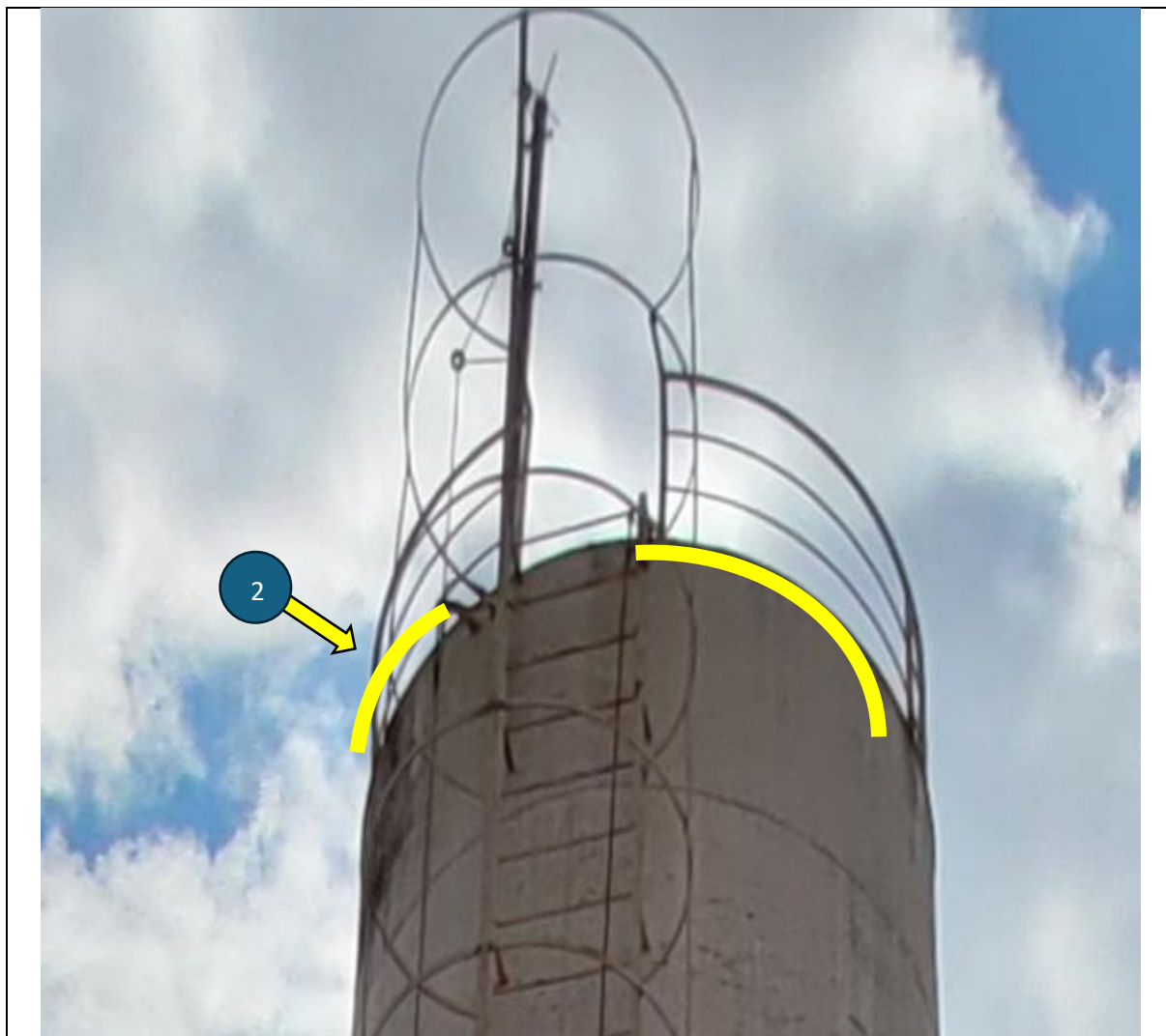
Figura 68 - Rodapé em torno do guarda corpo existente.
