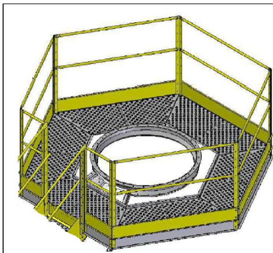
Imagem 78: Modelo de plataforma sextavada.
