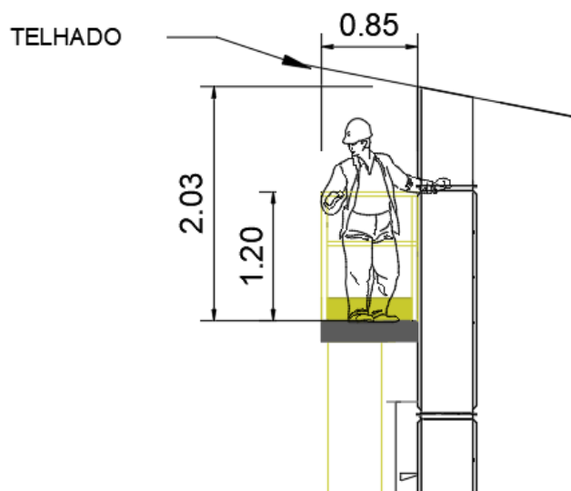
Figura 18 - Detalhe da plataforma a ser instalada
