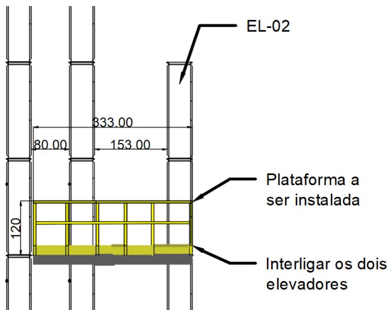
Figura 37 - Detalhe da plataforma a ser instalada interligando os dois elevadores.
