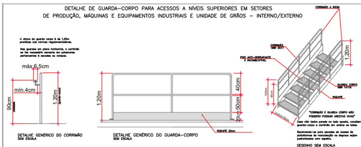
Imagem 72: Modelo construção de guarda corpo.
