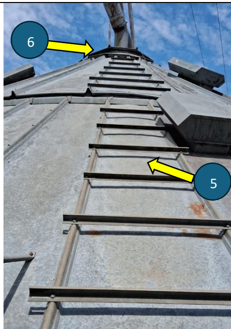
Figura 47 - Detalhe da adequação a ser realizada no telhado do silo pulmão.
