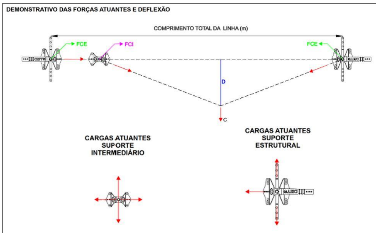
Imagem 92: Modelo do demonstrativo de esforços que deverá conter o documento final.
