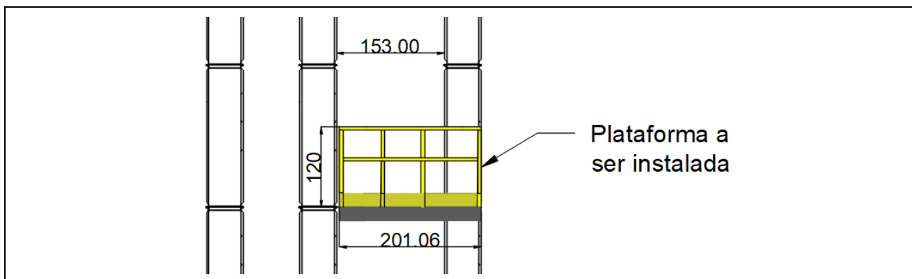
Figura 38 - Detalhe das plataformas a serem instaladas no elevador.
