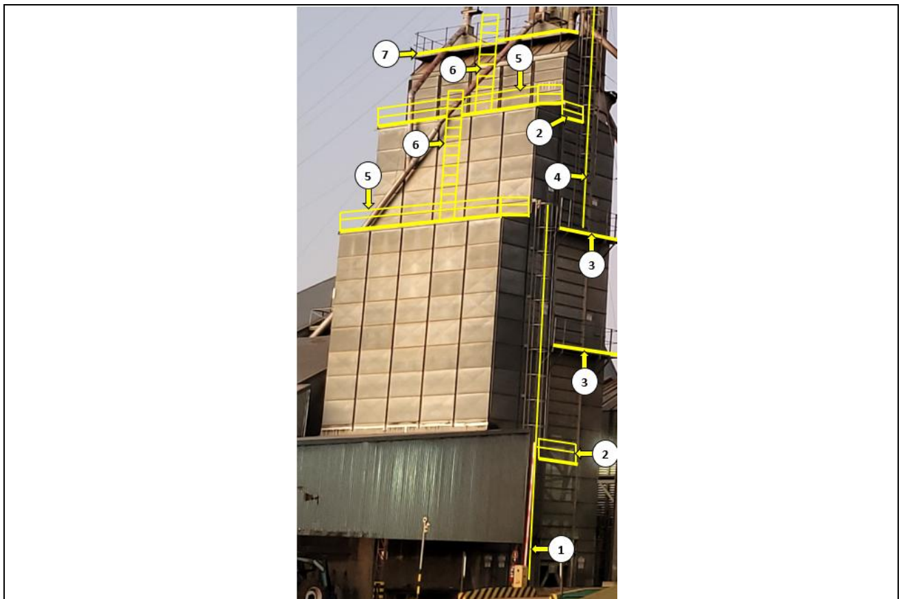
Figura 22 – Detalhe das adequações do secador.
