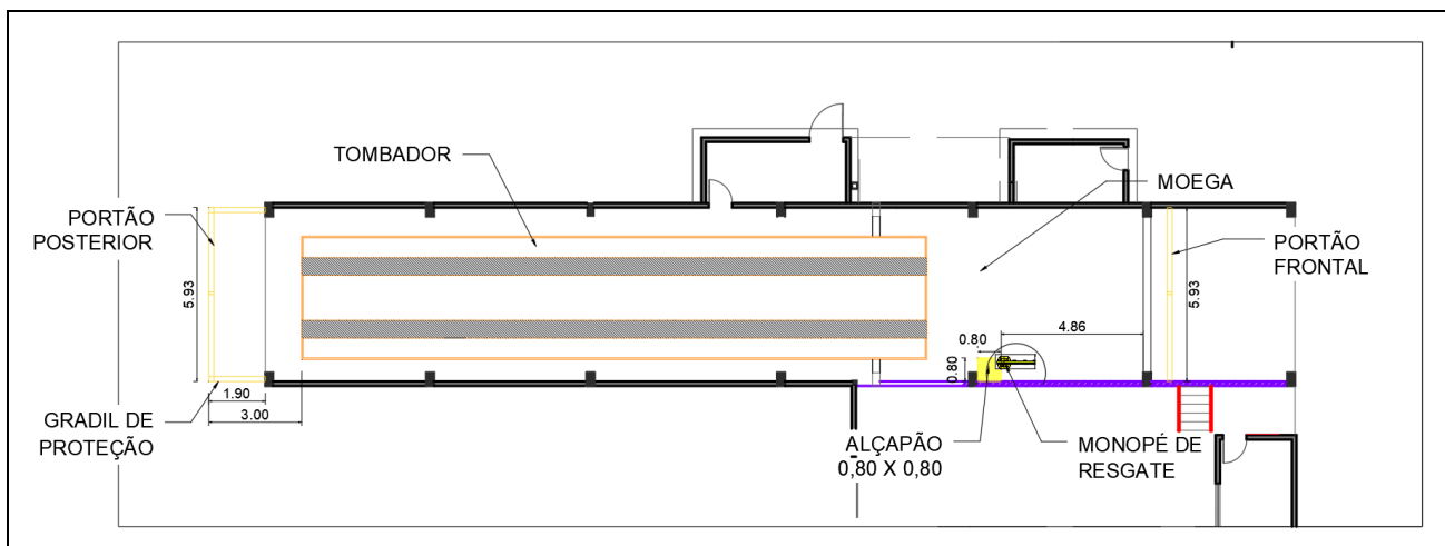
Figura 11 - Detalhe das adequações e medidas.
