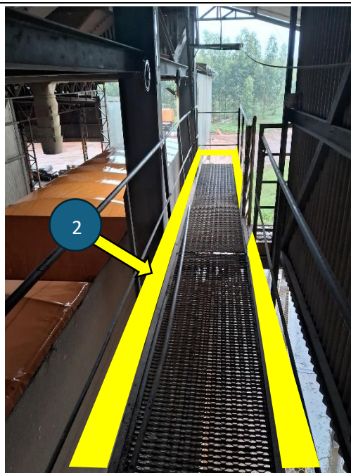
Figura 56 - Detalhe das adequações a serem realizadas.
