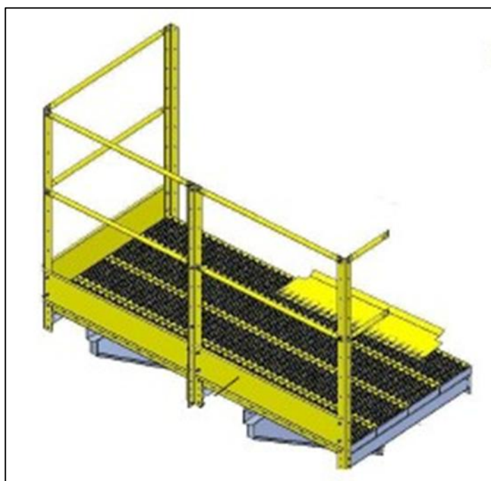
Imagem 73: Detalhe guarda corpo padrão.
