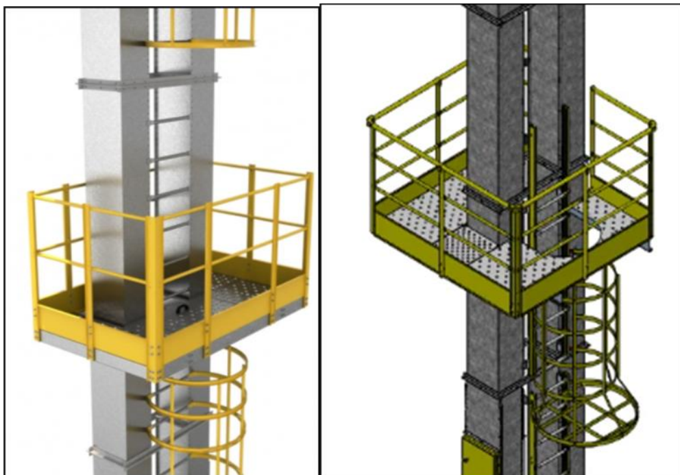
Imagem 83: Detalhe plataforma de fluxo contínuo.
