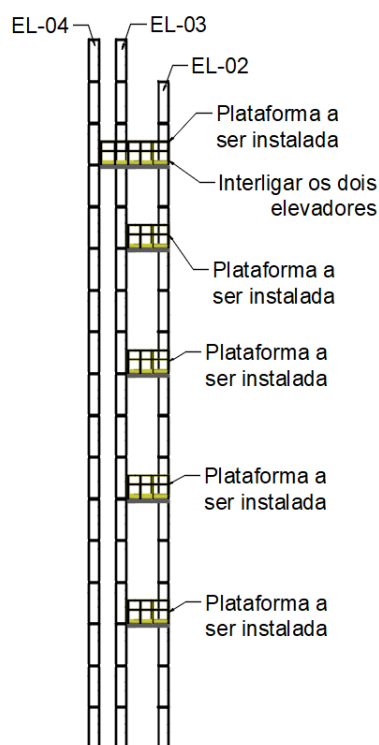
Figura 36 - Detalhe da adequação a ser realizada nos elevadores.
