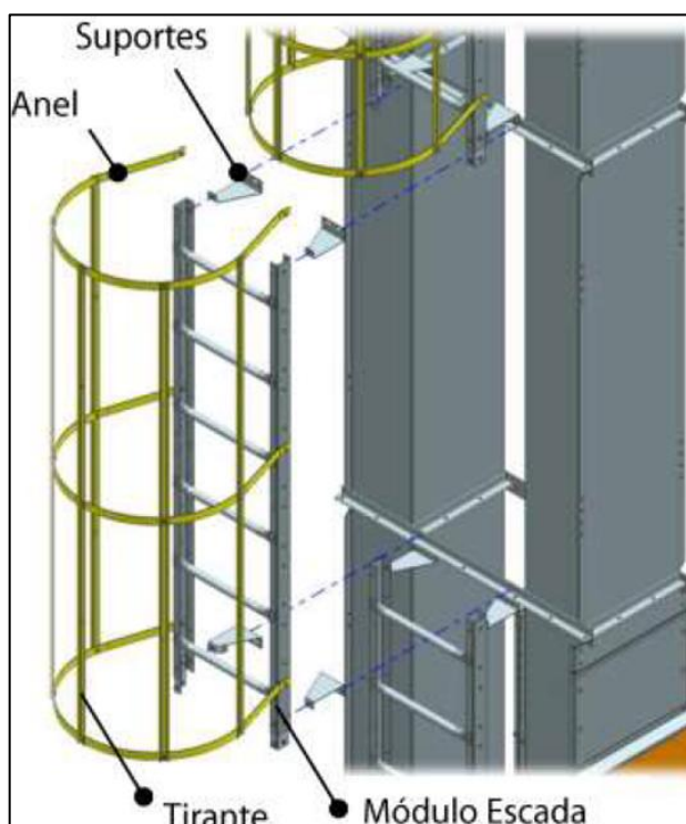
Imagem 80: Detalhes instalação da escada marinho com afastamento.
