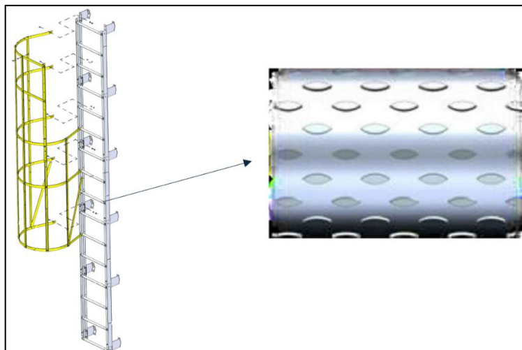
Imagem 79: Detalhes degrau antiderrapante da escada marinho.
