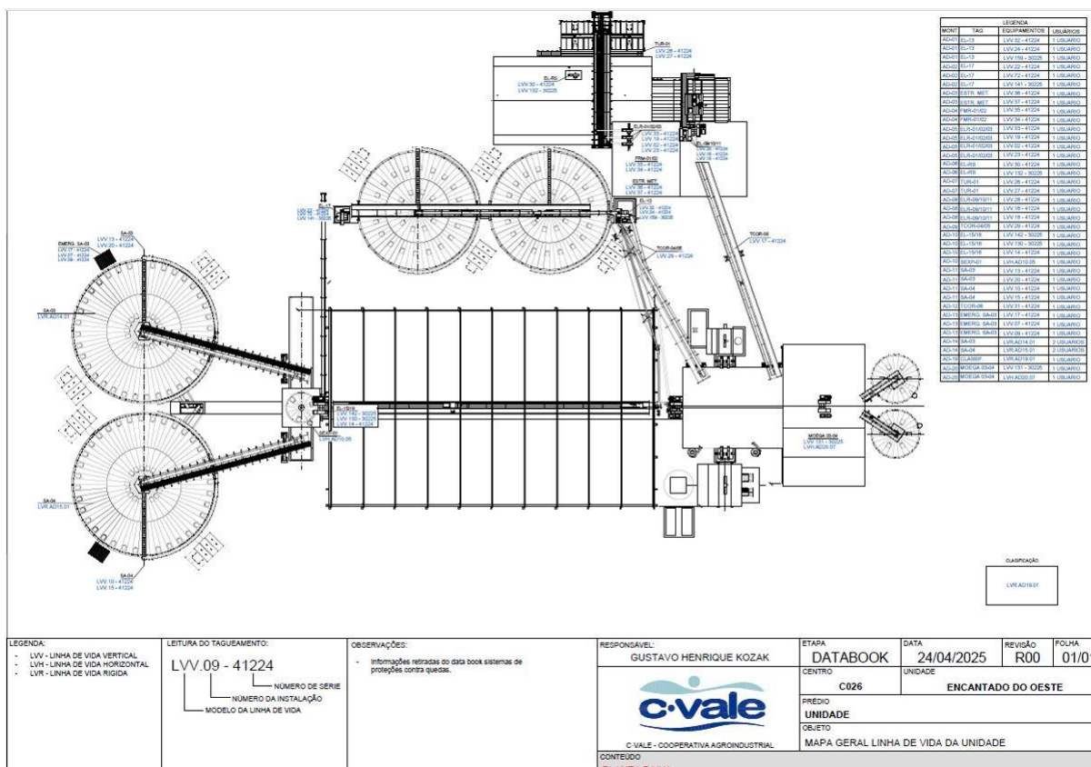
Imagem 93: Detalhe da planta baixa com as localizações das adequações e instalações das linhas de vida.
