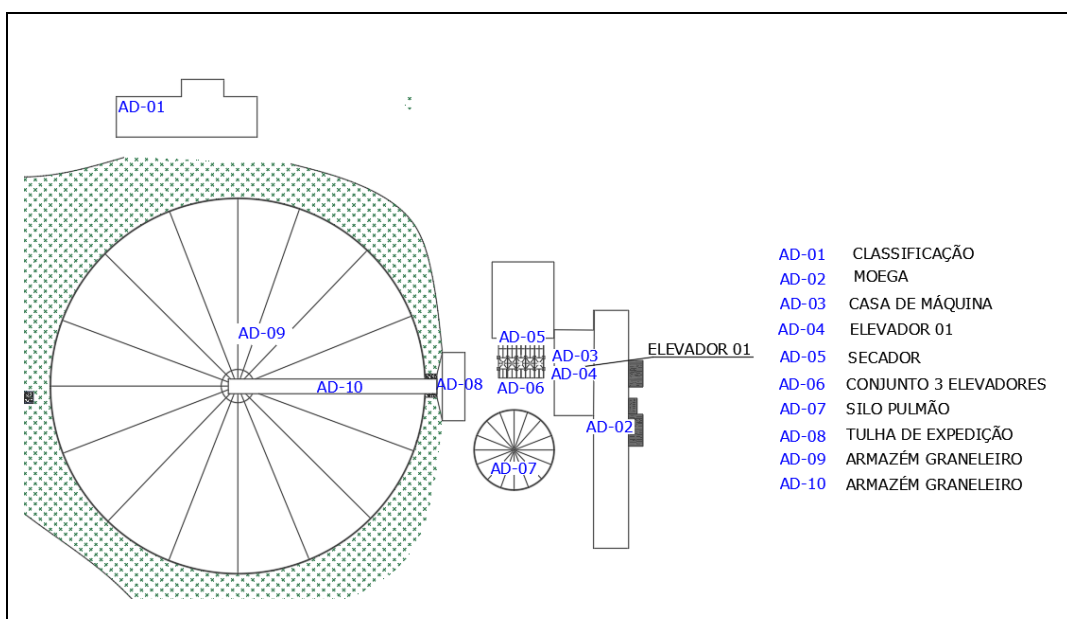
Figura 2 – Detalhe dos locais das instalações.
