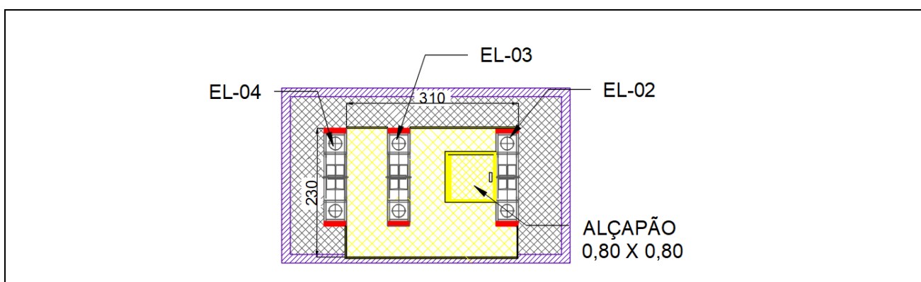
Figura 40 - Detalhes da plataforma interligando os dois elevadores.
