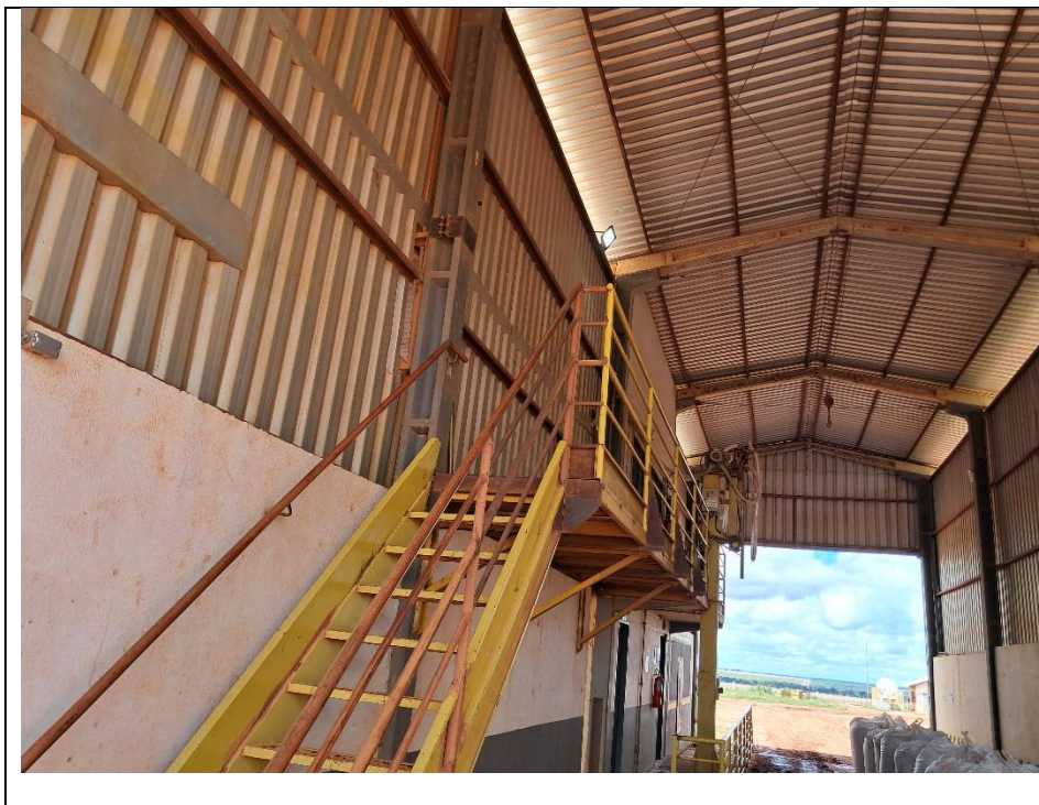
Figura 3 - Detalhe do prédio da classificação.
