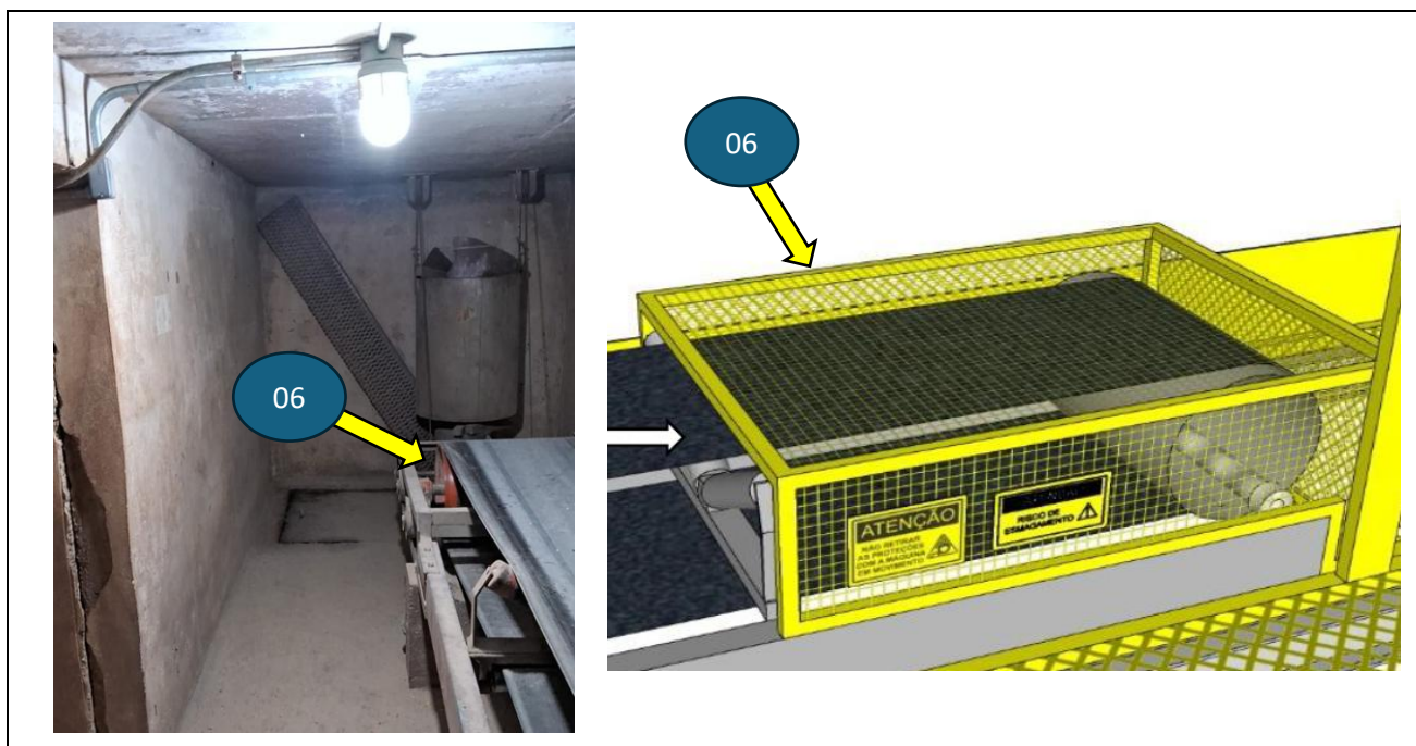
Figura 61 - Proteção para o movida da correia.
