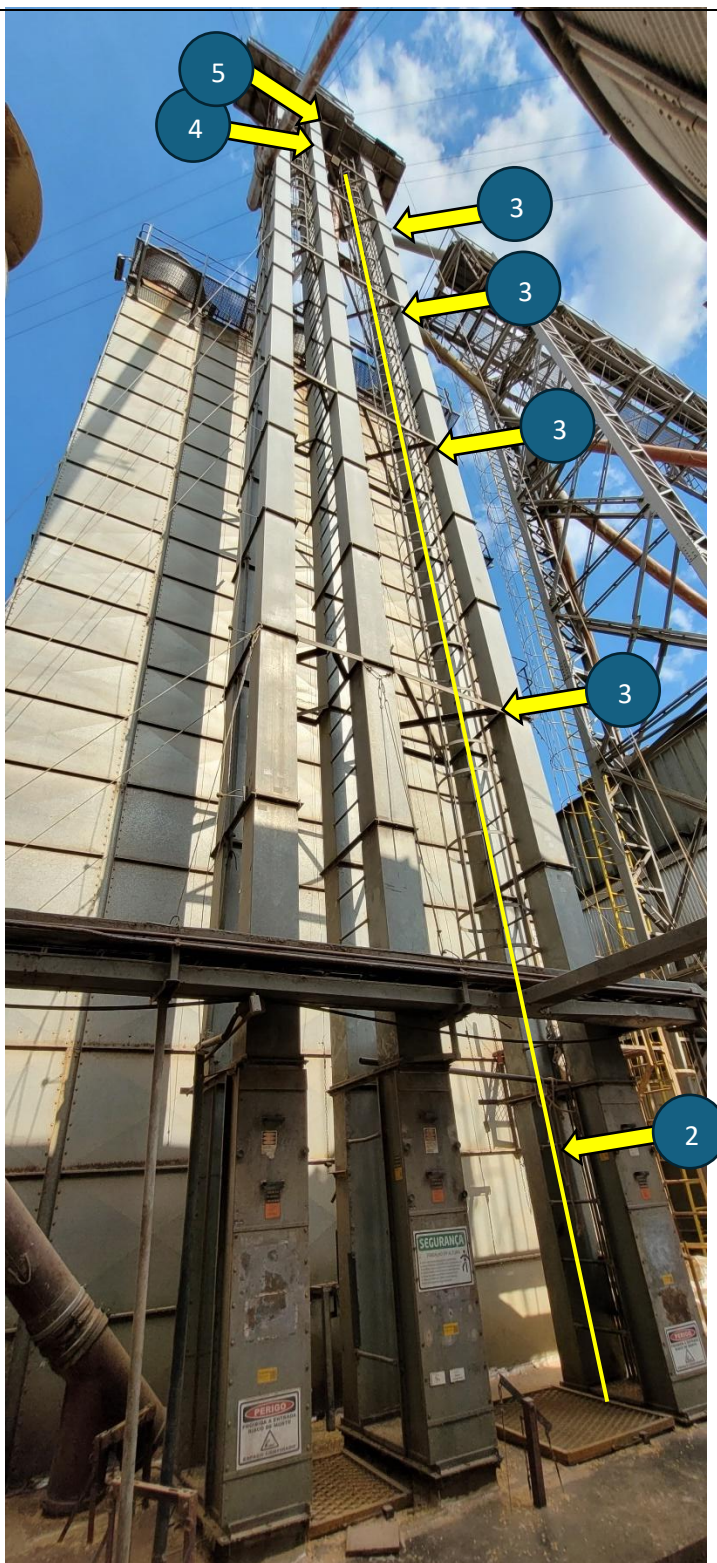
Figura 35 - Detalhe das adequações nos elevadores.
