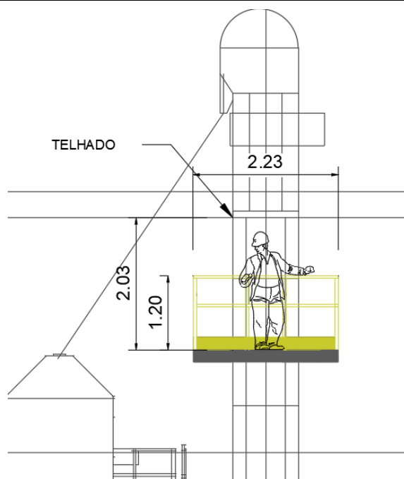
Figura 17 - Detalhe do local a instalar plataforma de descanso
