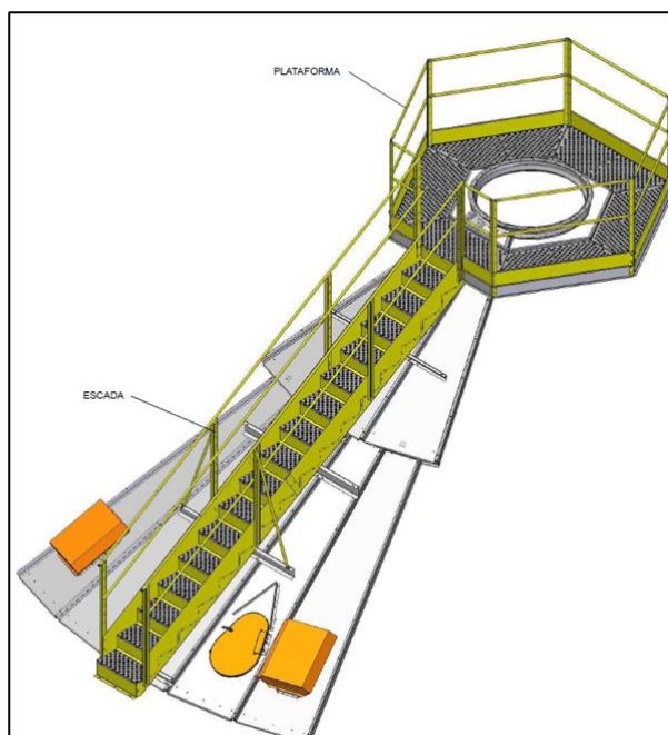
Imagem 77: Modelo de plataforma sextavada.
