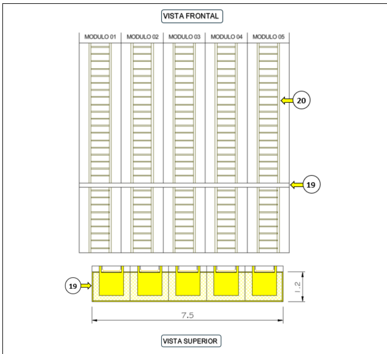
Figura 30 - Acesso interno C e D.
