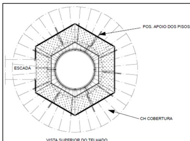
Imagem 76: Layout plataforma sextavada.
