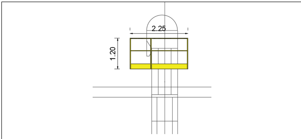
Figura 20 - Detalhe da plataforma a ser adequada
