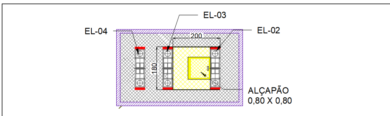
Figura 39 - Detalhe das 4 plataformas a serem instaladas.
