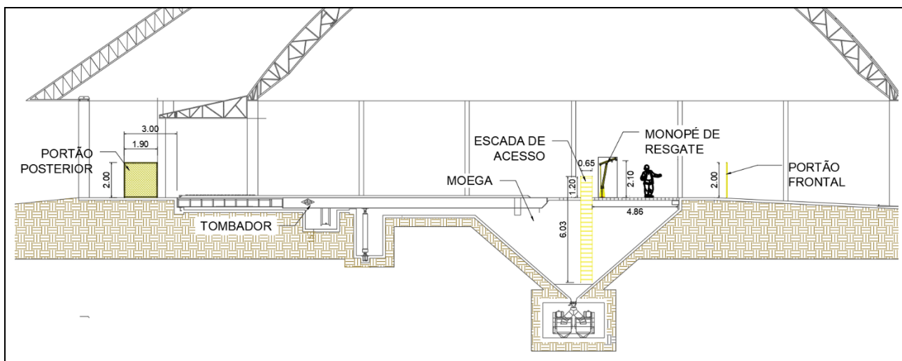
Figura 12 - Detalhe das adequações e medidas.
