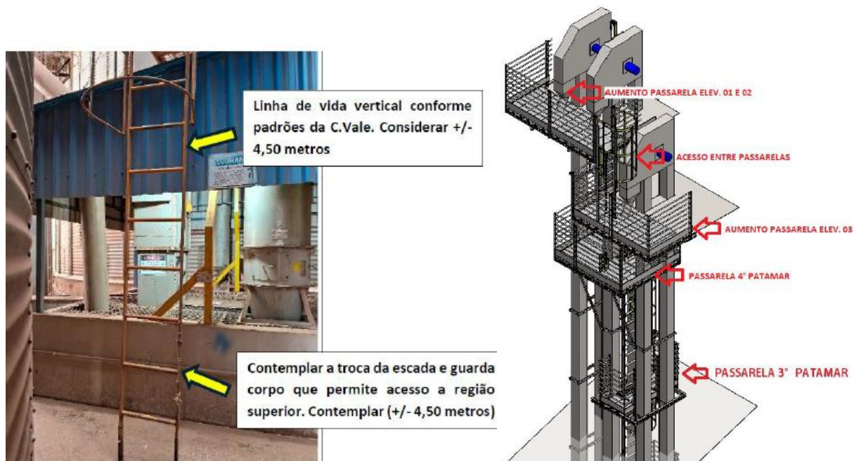
Imagem 88: Modelo de apresentação das adequações executadas, em relatório.
