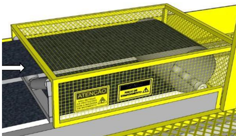
Figura 51 - Detalhe da proteção a instalar nos eixos da fita.
