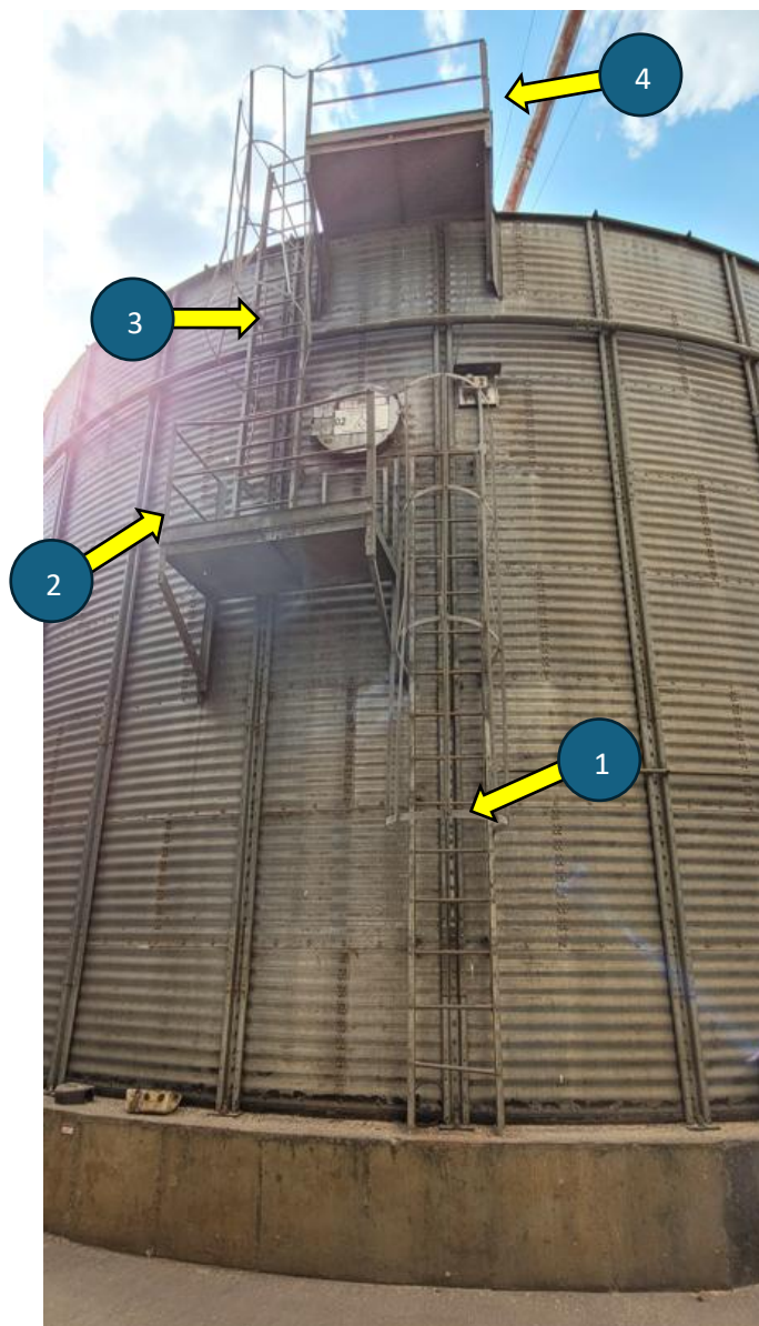
Figura 45 - Detalhe das adequações no silo pulmão.
