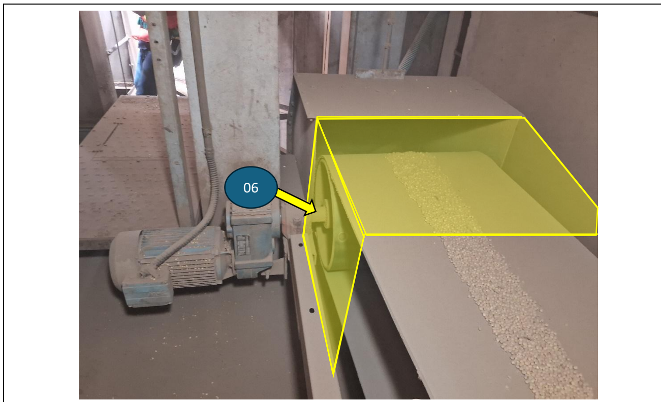
Figura 62 - Detalhe da proteção a ser instalado no chute da fita.
