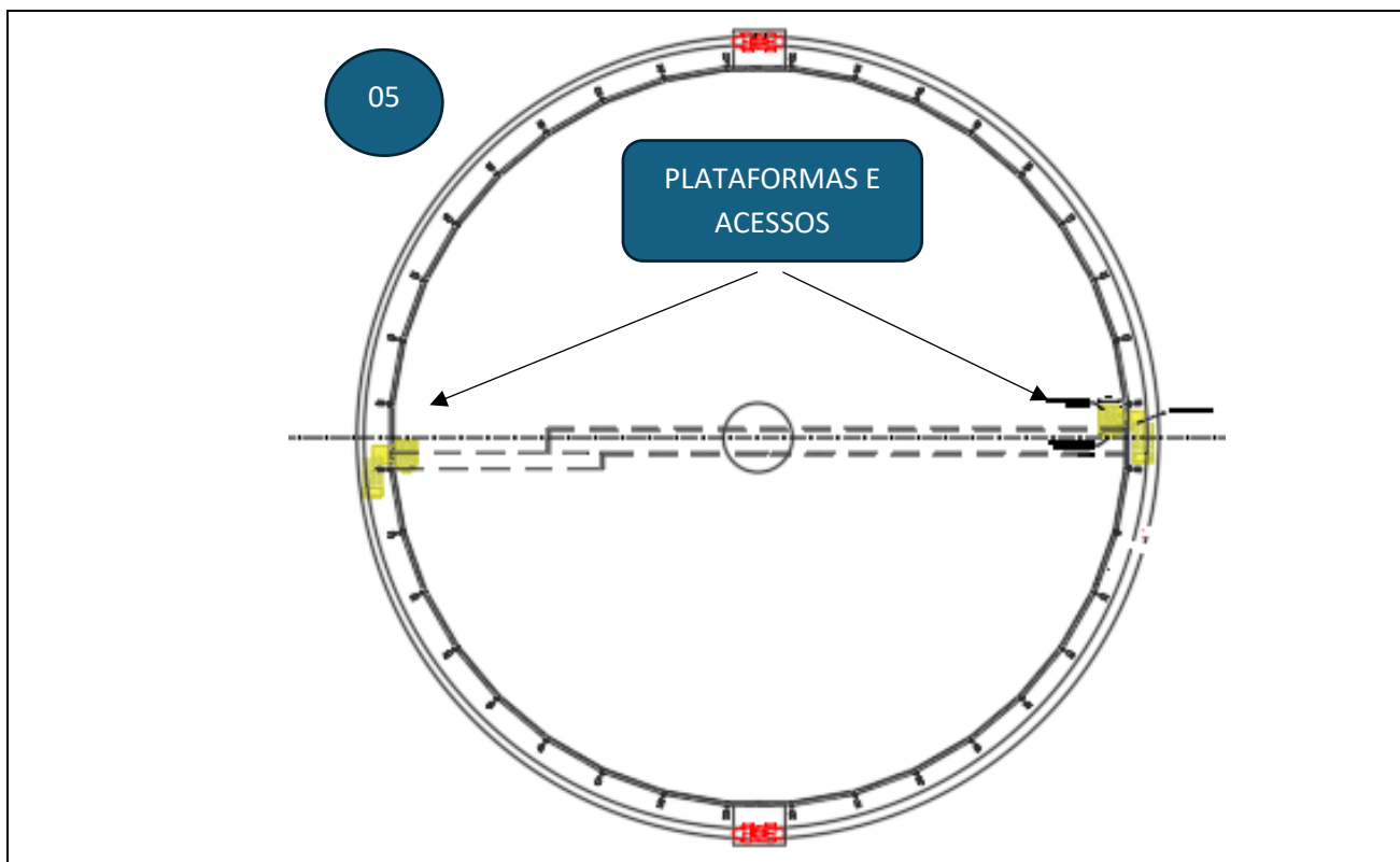
Figura 60 - Detalhe dos acessos a serem instalados.
