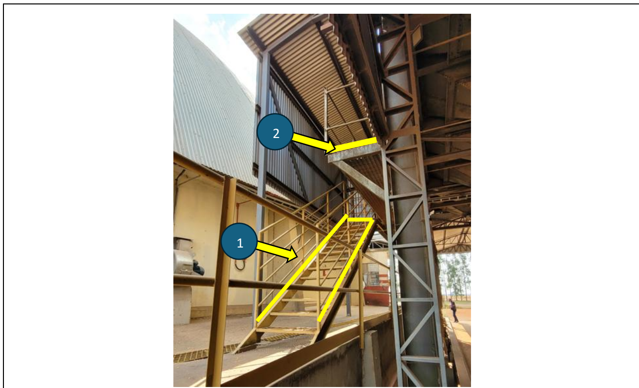
Figura 53 - Detalhe das adequações a serem realizadas na tulha.
