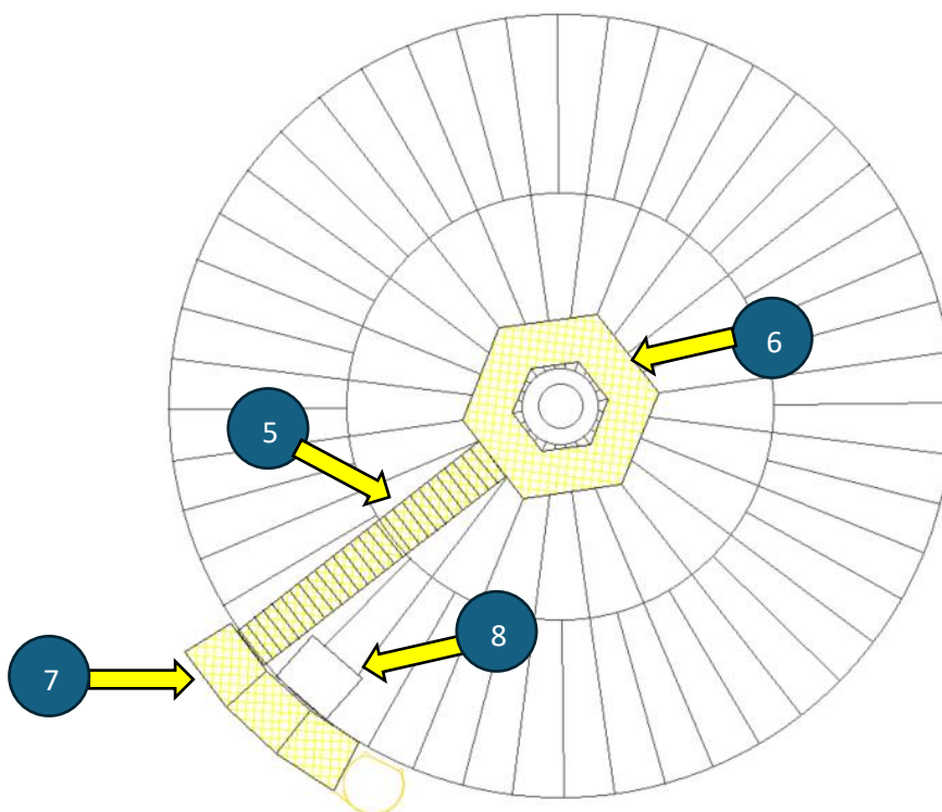
Figura 49 - Detalhe da adequação a ser realizada no silo pulmão.
