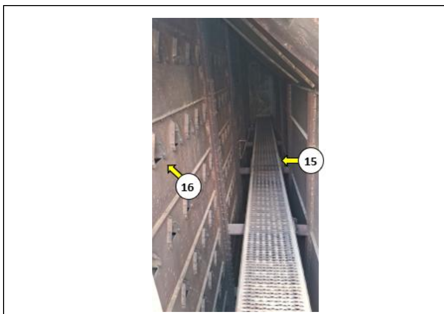
Figura 29 - Acesso interno B.
