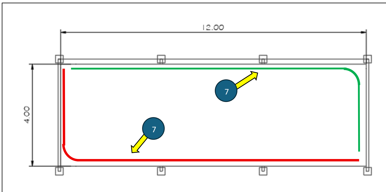
Figura 59 - Detalhe das linhas de vida a serem instaladas.
