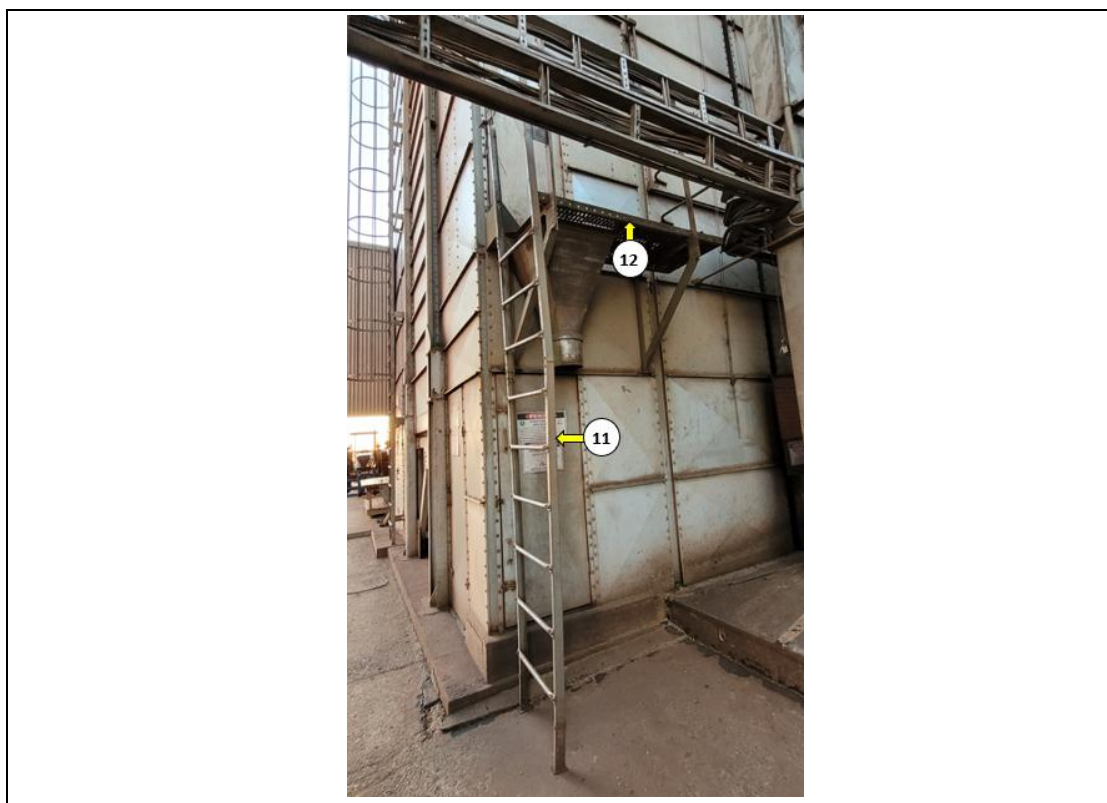
Figura 25 - Detalhe das adequações a serem realizadas no secador.
